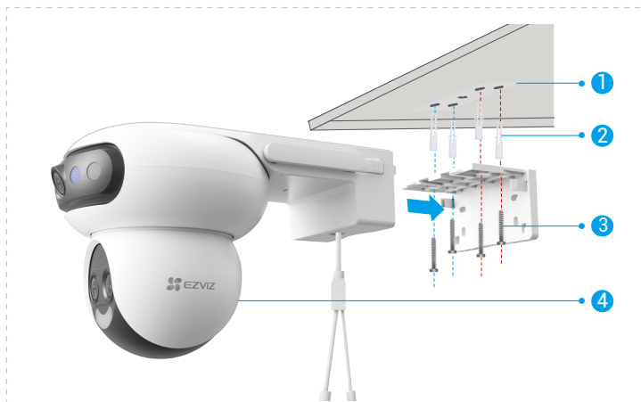
Fig. 1 Takmontering
