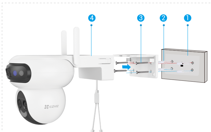
Fig. 2 Väggmontering
